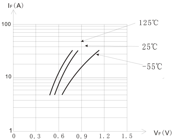
图 2 V_F-I_F 特性曲线
