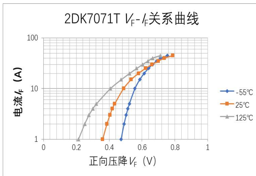
图 2 V_F-I_F 特性曲线
