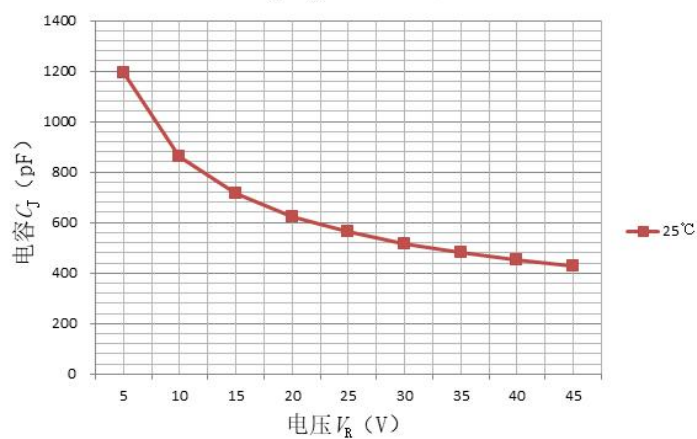
图3 C_J - V_R 特性曲线
