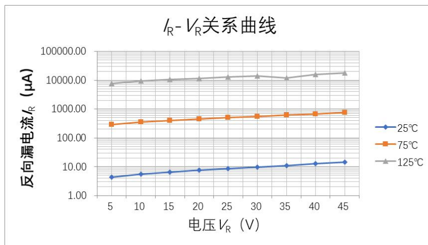
图 1 I_R-V_R 特性曲线
