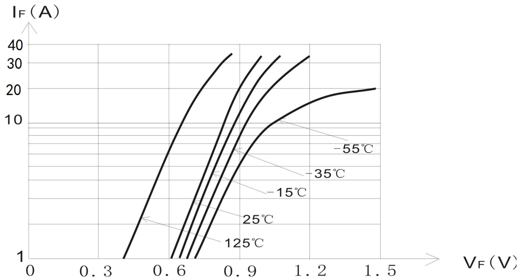
图2 V_F-I_F 特性曲线
