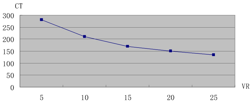
图 3 C_T-V_R 特性曲线
