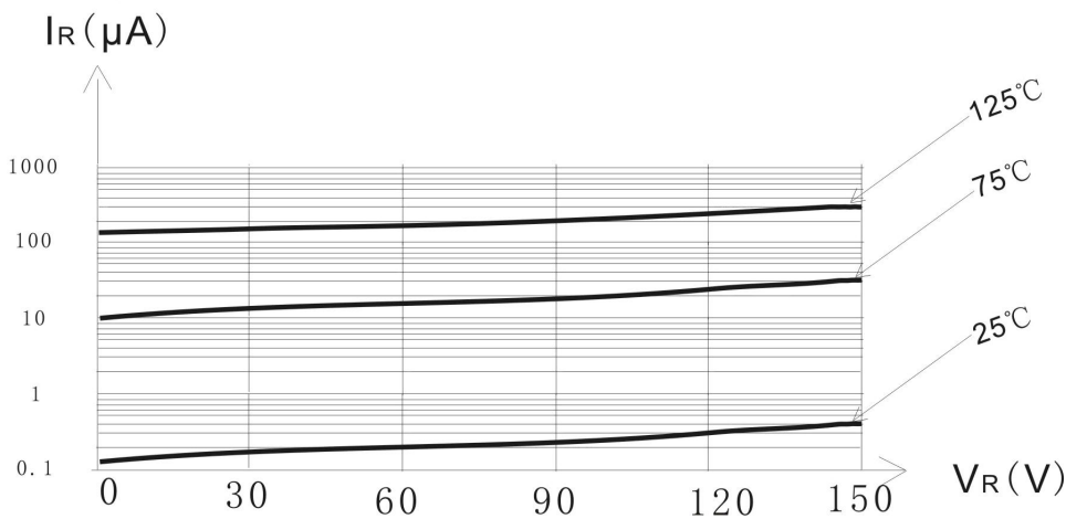
图 1 I_R — V_R 特性曲线
