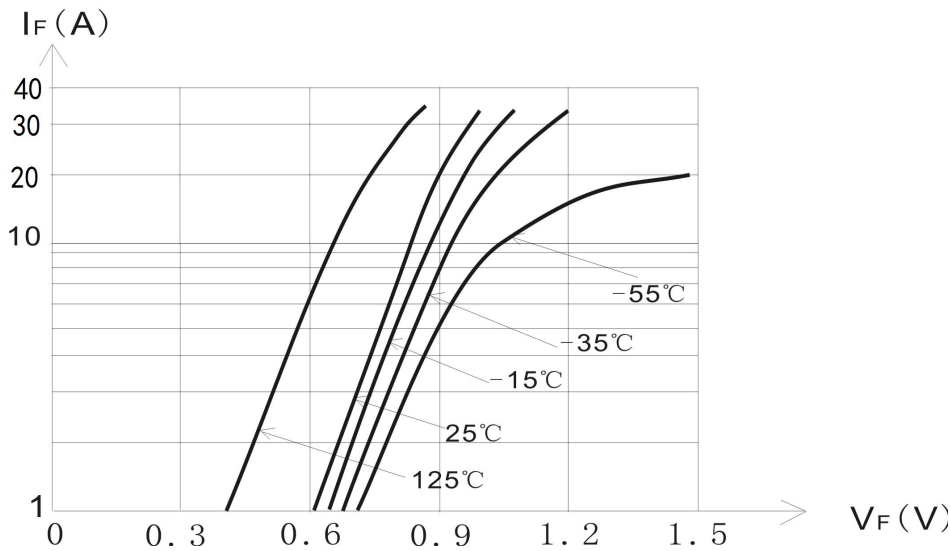
图 2 V_F — I_F 特性曲线
