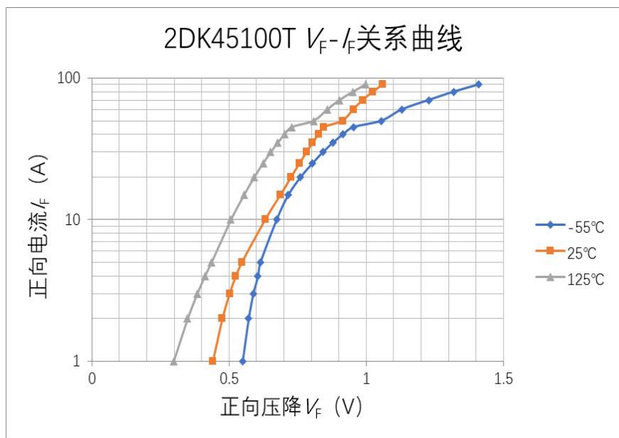
图2 V_F-I_F 特性曲线
