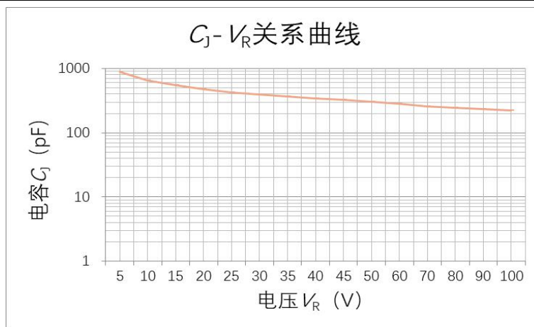
图 3 C_J - V_R 特性曲线
