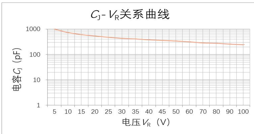
图 3 C_{tot} — V_R 特性曲线
