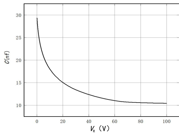
图3 结电容特性曲线
