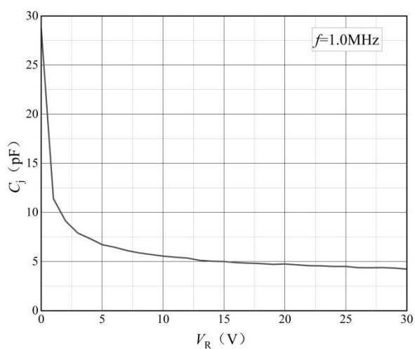
图3 结电容特性曲线
