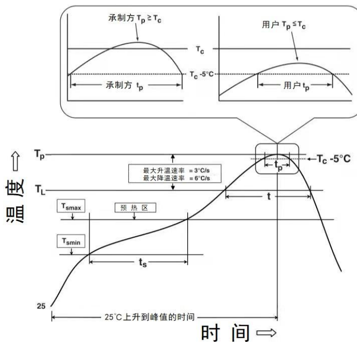
图 10 回流温度-时间分布图
