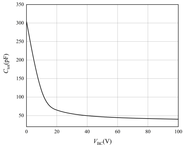
图 5 电容-电压特性曲线
