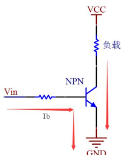
图 7 典型开关电路原理图
