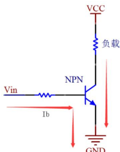
图 6 典型开关电路原理图
