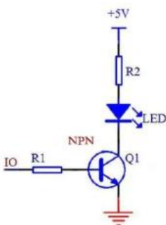
图 7 典型电流放大电路原理图
