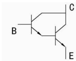
图 8 达林顿管 NPN 结构原理图
