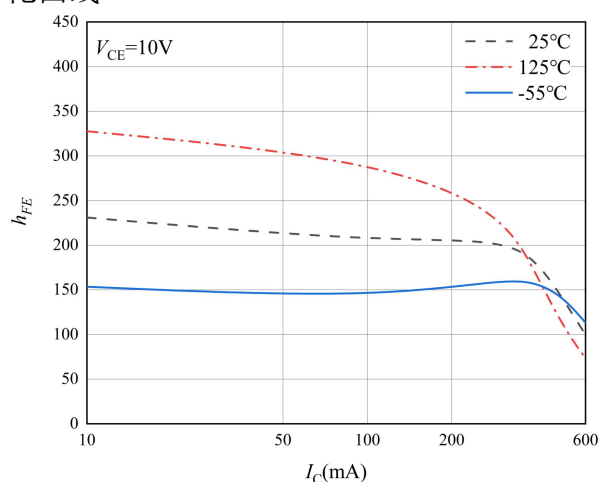
图 2 直流电流增益特性曲线
