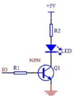
图 7 典型电流放大电路原理图
