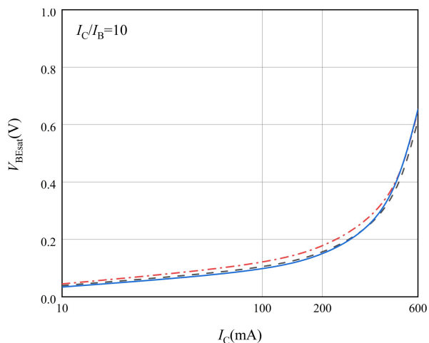
图 3 CE 端饱和和压降特性曲线
