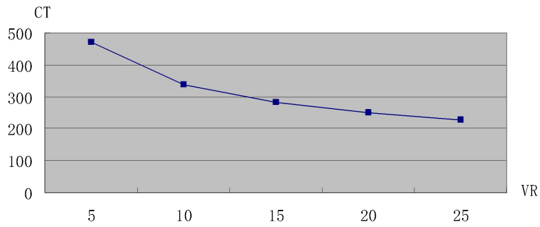
图 3 C_{tot} — V_R 特性曲线
