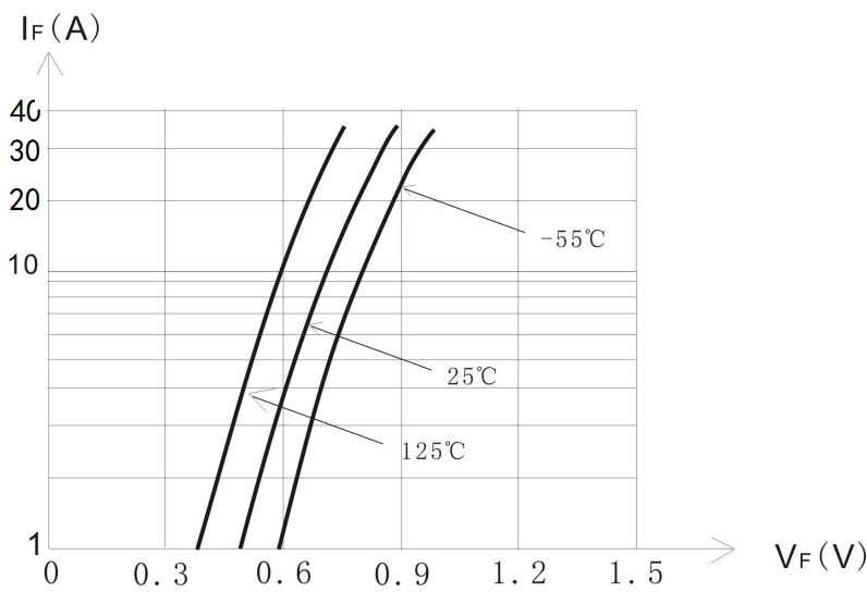
图 2 V_F-I_F 特性曲线
