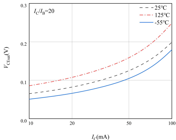
图 4 CE 端饱和压降特性曲线
