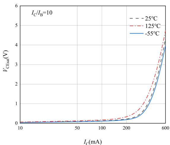
图 3 CE 端饱和压降特性曲线
