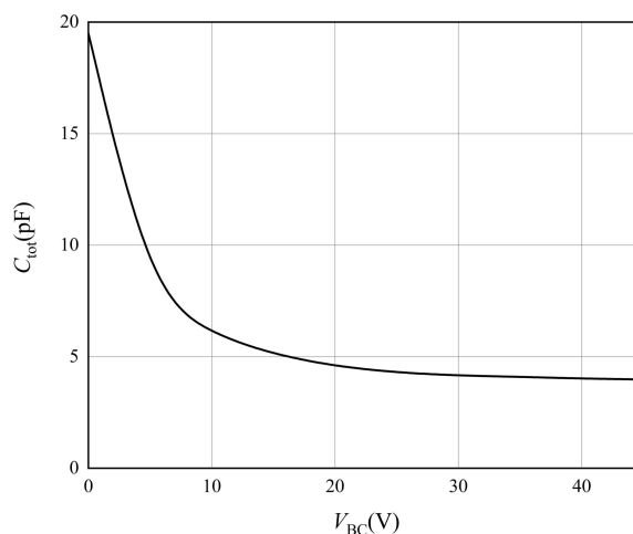
图 2 电容-电压特性曲线
