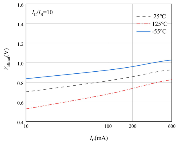
图 4 BE 端饱和压降特性曲线
