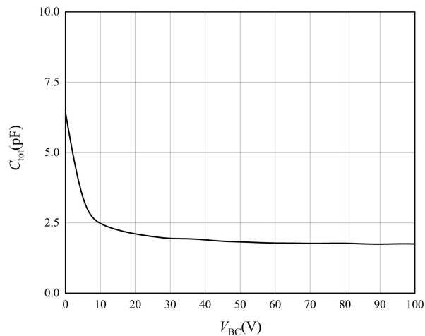
图 2 电容-电压特性曲线
