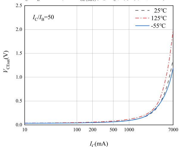
图 5 CE 端饱和压降特性曲线
