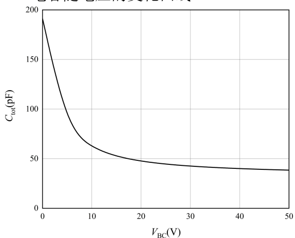
图 7 电容-电压特性曲线
