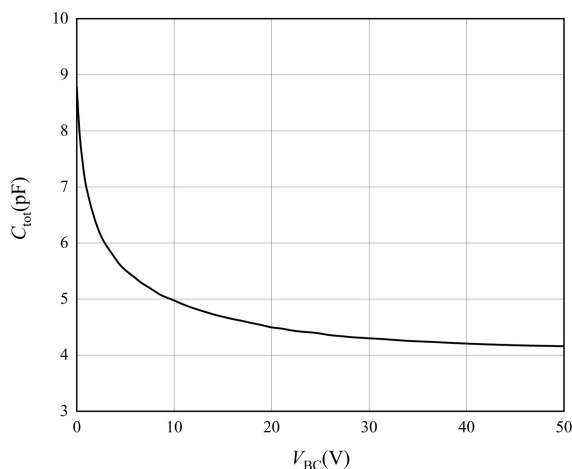
图 2 电容-电压特性曲线
