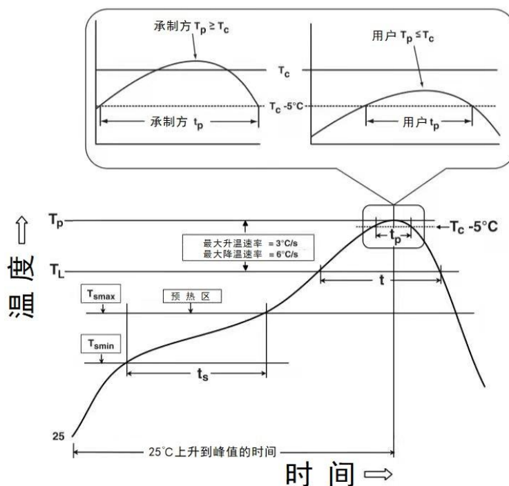
图 13 回流温度-时间分布图
