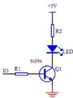
图 11 典型电流放大电路原理图
