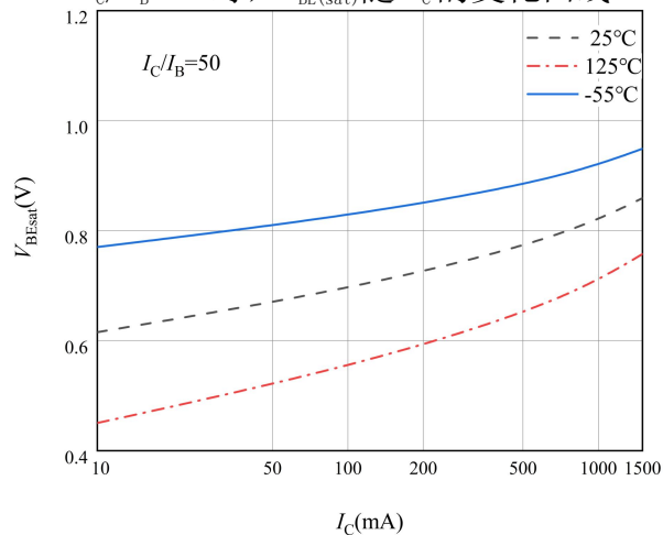
图 8 BE 端饱和和压降特性曲线
