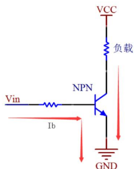
图 10 典型开关电路原理图
