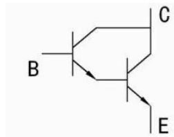
图 12 达林顿管 NPN 结构原理图
