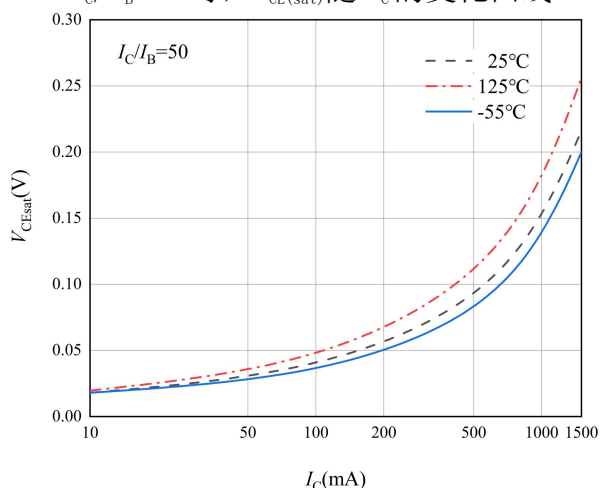
图 7 CE 端饱和和压降特性曲线
