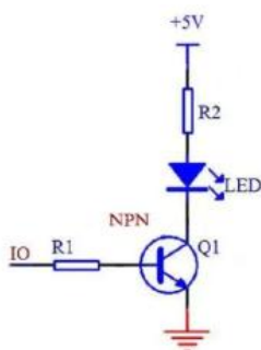
图 8 典型电流放大电路原理图
