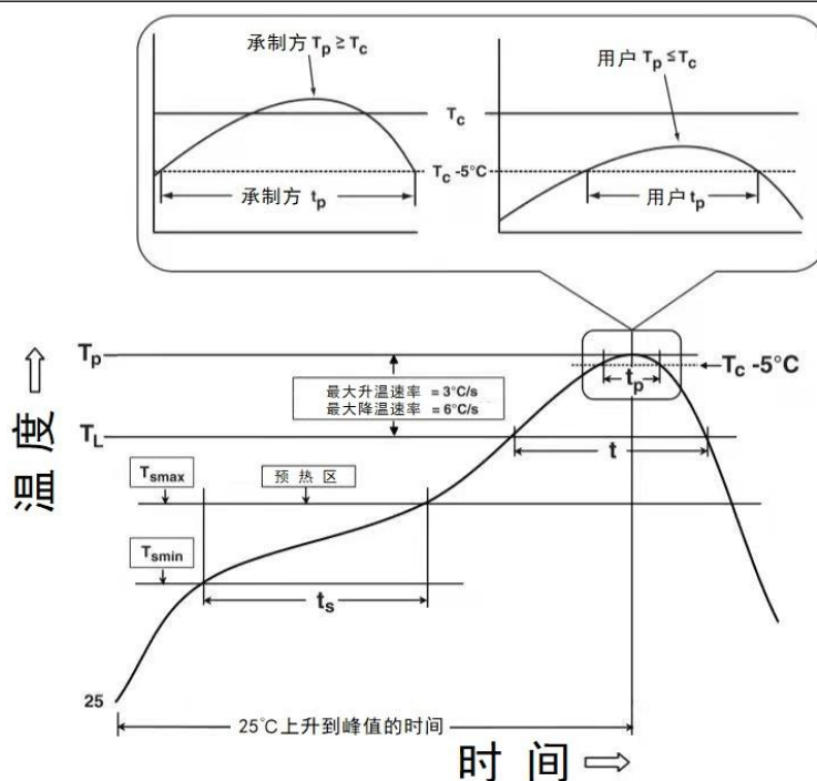
图 10 回流温度-时间分布图
