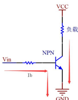
图 7 典型开关电路原理图
