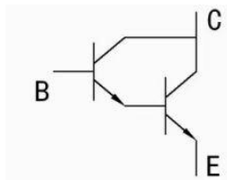
图 9 达林顿管 NPN 结构原理图
