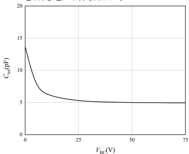
图 5 电容-电压特性曲线
