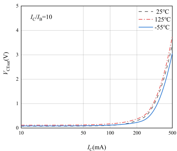
图 3 CE 端饱和和压降特性曲线
