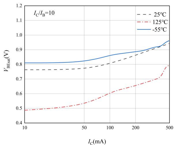
图 4 BE 端饱和和压降特性曲线
