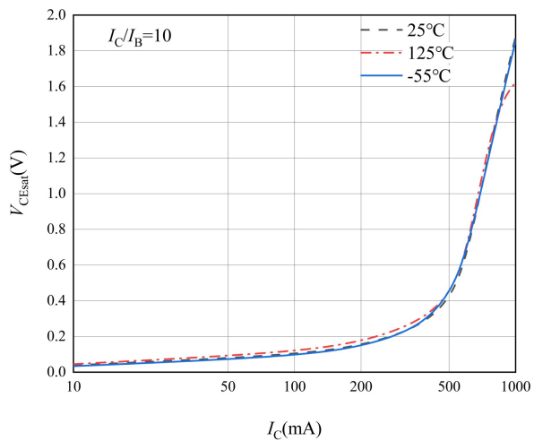
图 3 CE 端饱和压降特性曲线 7.5 电容随电压的变化曲线
