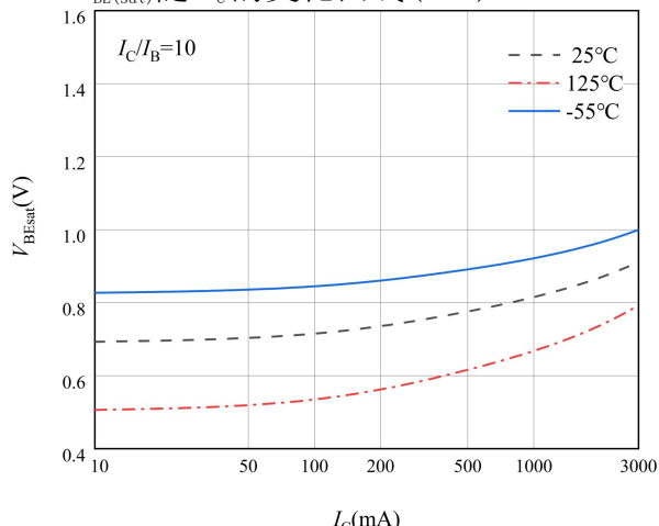
图 8 BE 端饱和和压降特性曲线
