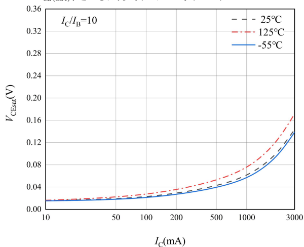
图 6 CE 端饱和和压降特性曲线
