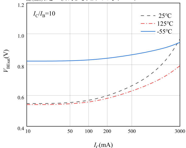
图 7 BE 端饱和和压降特性曲线
