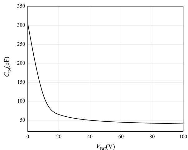
图 10 电容-电压特性曲线
