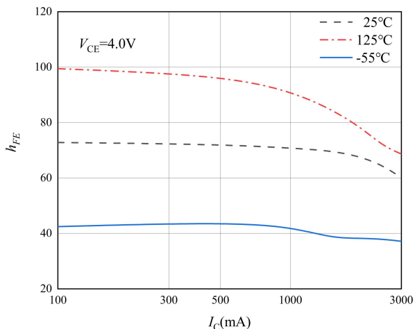
图 3 直流电流增益特性曲线
