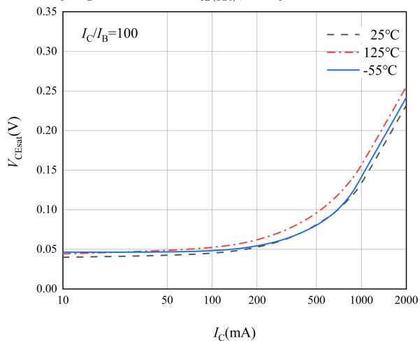
图 5 CE 端饱和和压降特性曲线
