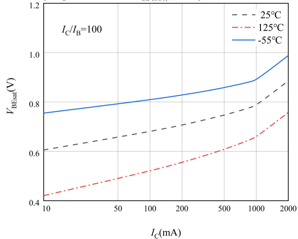
图 6 BE 端饱和和压降特性曲线
