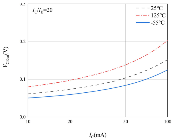
图 3 CE 端饱和压降特性曲线
