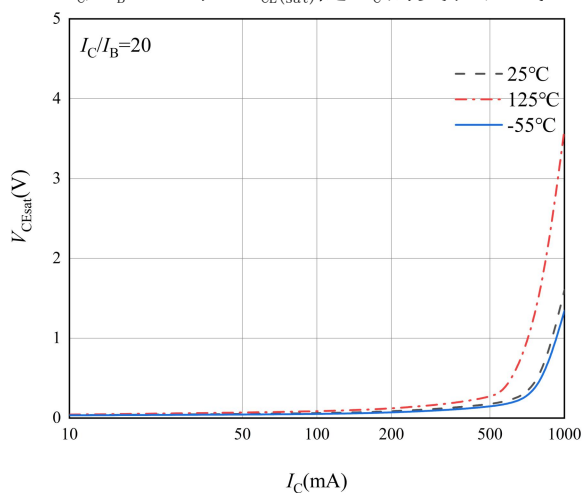
图 5 CE 端饱和和压降特性曲线
