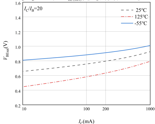
图 6 BE 端饱和和压降特性曲线
