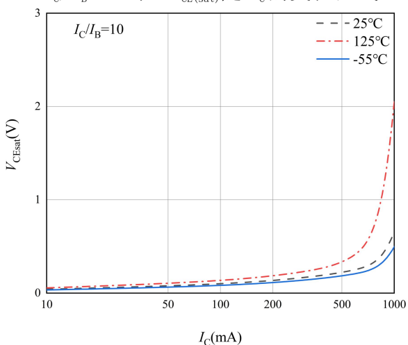
图 7 CE 端饱和和压降特性曲线
