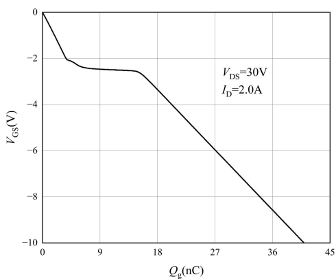
图 9 PMOS- V_{GS} - Q_g 特性曲线
