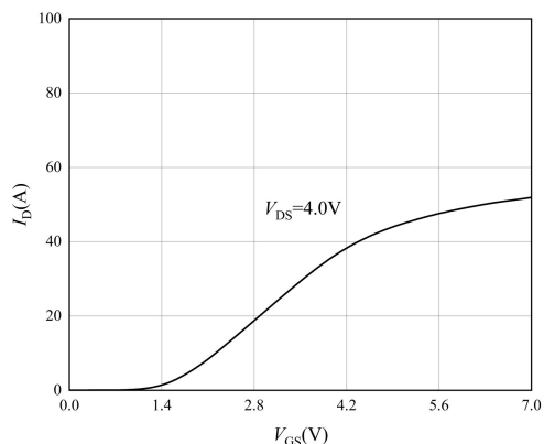
图 7 PMOS 转移特性曲线
