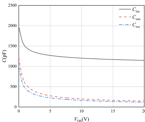
图 5 NMOS- C - V_{DS} 特性曲线
