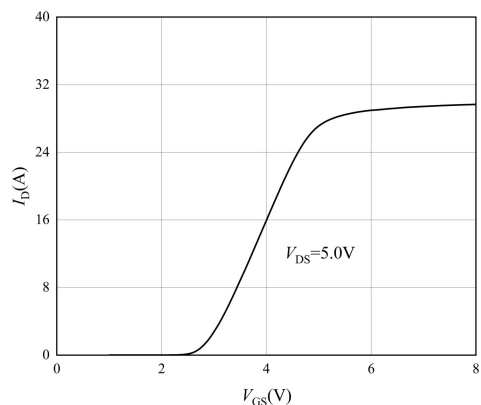
图 7 PMOS 转移特性曲线
