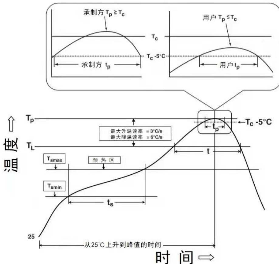
图 5 回流温度-时间分布图
