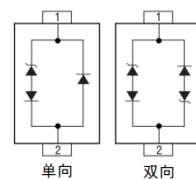
电原理图
