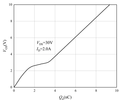
图 4 V_{DS}-Q_g 特性曲线
