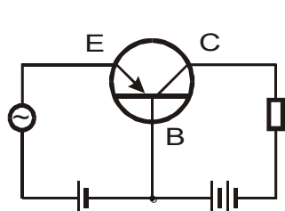
共基极接线法
