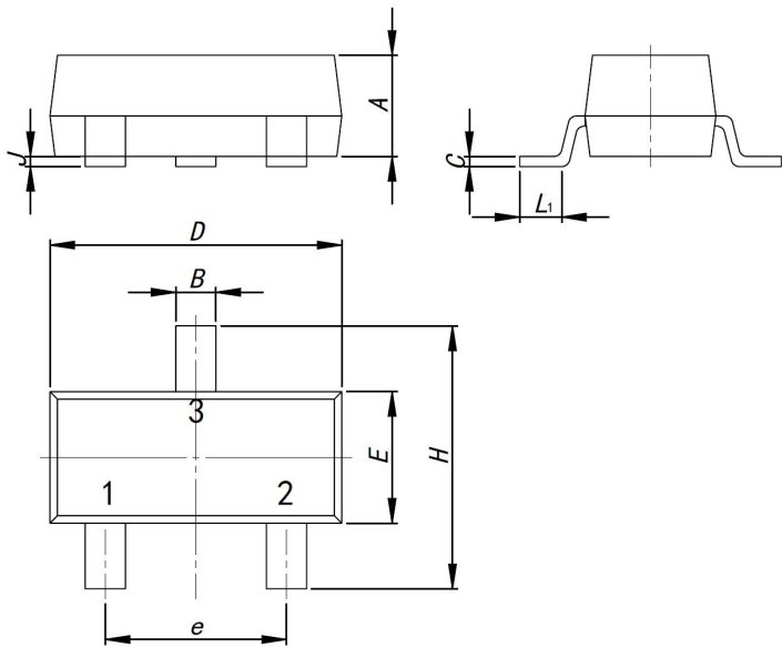
引出端：1-栅极 G，2-源极 S，3-漏极 D
