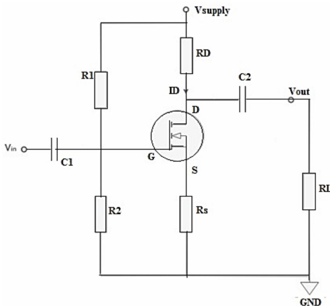
图 8 典型放大电路
