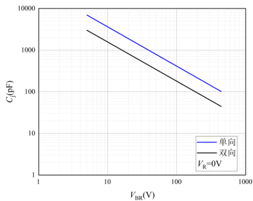
图 3 电容曲线
