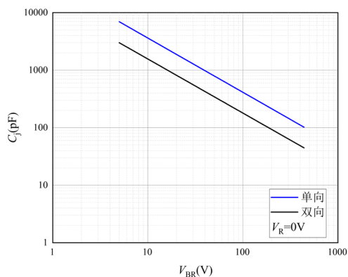
图 3 电容曲线
