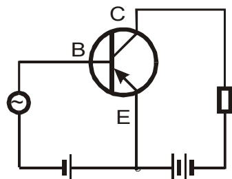
共发射极接线法
