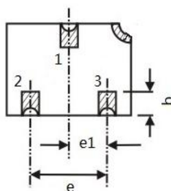
SMD-0.2 外形尺寸
