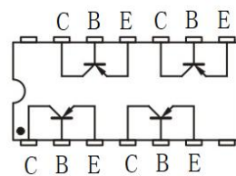
T型
