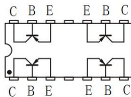
S型
