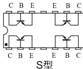
DIP-14 型双列直插陶瓷封装
