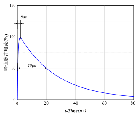
图 2 8/20 脉冲波形曲线
