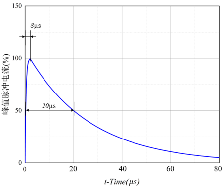
图 2 8/20 脉冲波形曲线
