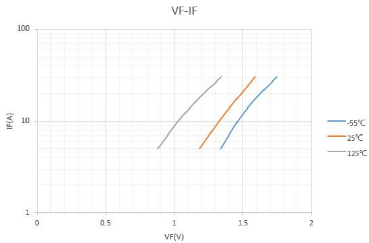
图2 V_F-I_F 特性曲线
