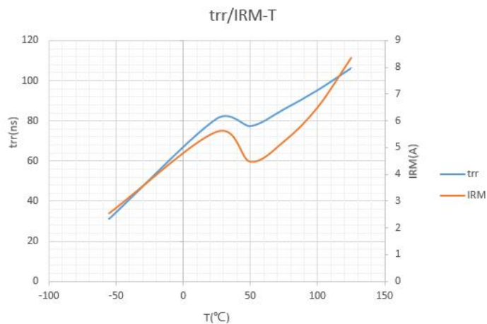
图 3 t_{rr}/I_{RM} -T 特性曲线
