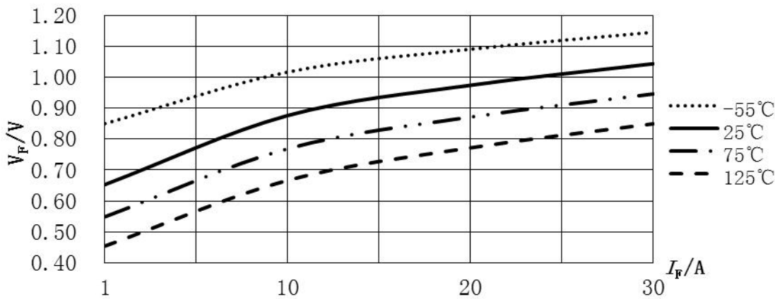
图 2 V_F-I_F 特性曲线
