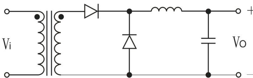
图 7 整流加续流电路
