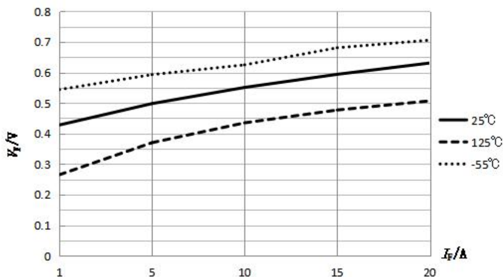
图 2 V_F - I_F 特性曲线
