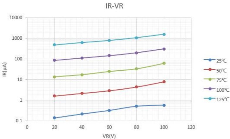
图 1 I_R-V_R 特性曲线
