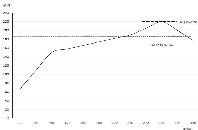
图 7 建议的回流焊曲线
