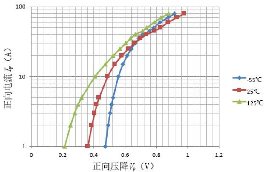
图2 V_F - I_F 特性曲线
