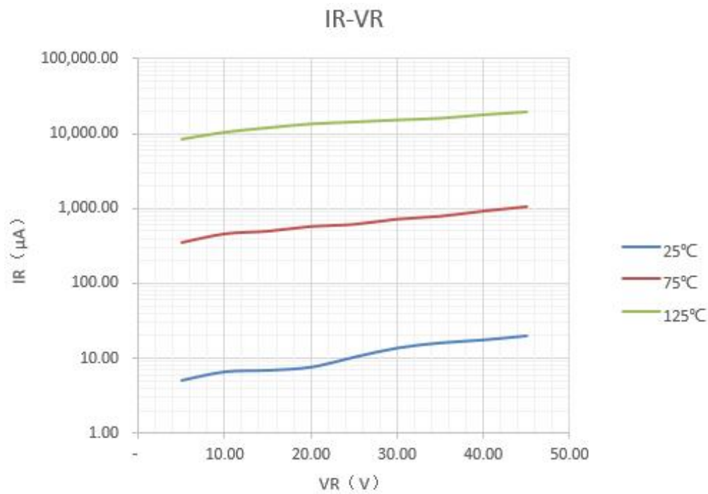
图 1 I_R-V_R 特性曲线
